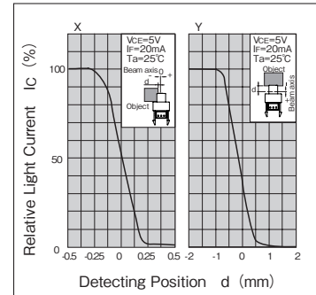
検出位置特性 (代表例)
