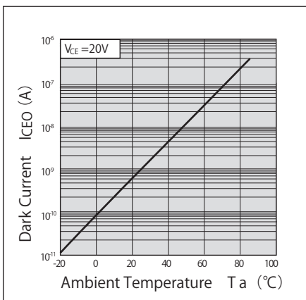
暗電流一周圍温度特性 (代表例)
